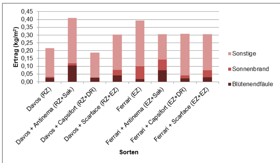
Abb. 2: Nicht marktfähige Paprika-Erträge pro m 2 beim Anbau im kalten Folienhaus
