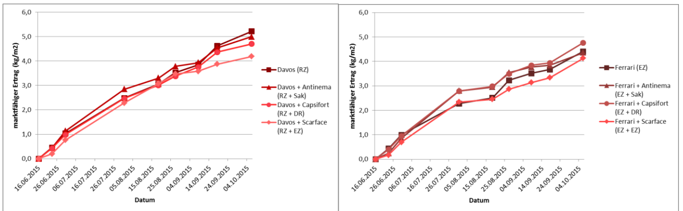
Abb. 1: Marktfähiger Paprika-Ertrag pro m 2 im Ernteverlauf beim Anbau im kalten Folienhaus.
